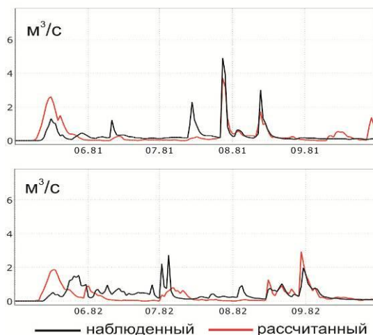
Рис. 5. Рассчитанный и наблюдаемый гидрограф стока (м 3 /с), ручей Контактный, 1981-1982 гг.
