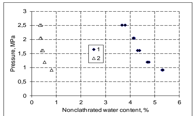
Рис. 4. Изменение содержания неклатратной воды в зависимости от давления CO_2 в модельных грунтах при -7.5^\circ C . 1- песок с 25% частиц монтмориллонитовой глины и 2- песок с 25% частиц каолиновой глины
