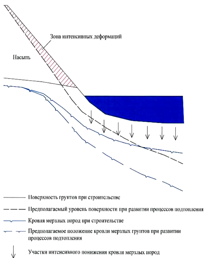
Рис. 6. Развитие деформаций из-за увеличения крутизны откоса насыпи в результате подтопления
