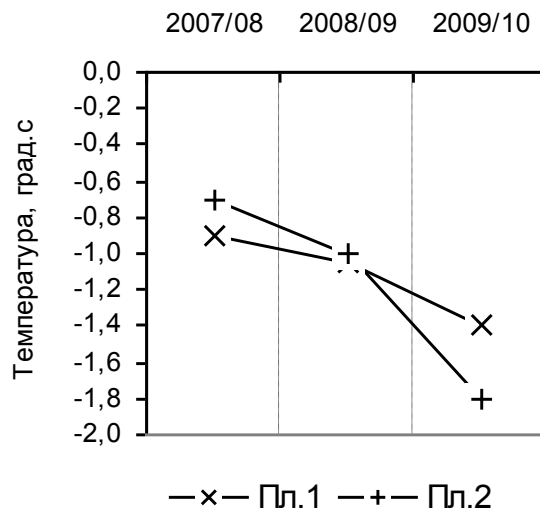
Рис.5. Средние годовые температуры грунта на глубине 3.2 м.
