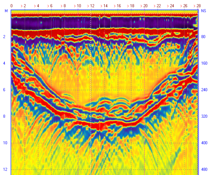
Рис. 6 Радарограмма Сусловской воронки.
