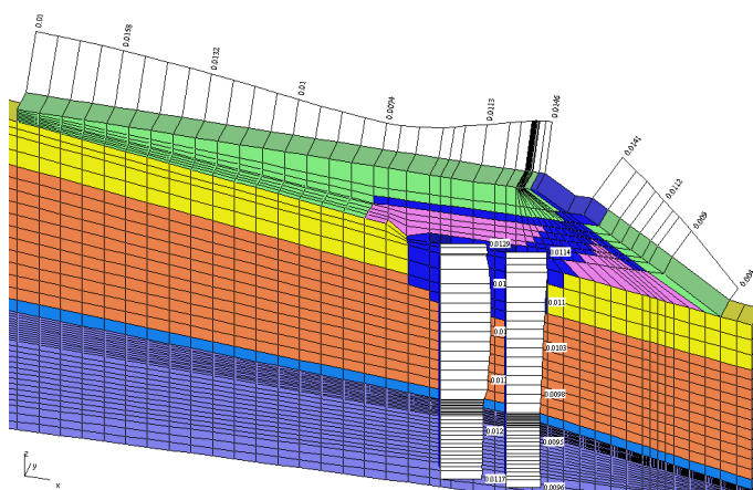
Рис. 4. Эпюры горизонтальных перемещений элементов свайно-ростверковой конструкции, м
