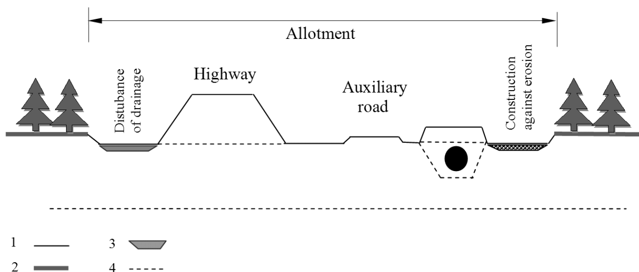
Рис 2. Обобщённый поперечный профиль коридора магистрального нефтепровода: 1 – незадернованная поверхность; 2 – задернованная поверхность; 3 – водоём; 4 – литологическая граница
