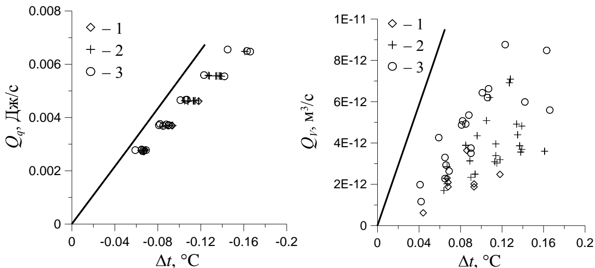
Рис. 4. Потоки тепла (а) и вещества (б) через образец в зависимости от разности температур на его основаниях. Символы - экспериментальные данные при различных средних температурах t_0 [°C]: -0,04 (1); -0,03 (2); -0,02 (3). Линии – результат расчета
