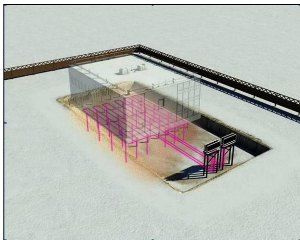
Рис. 5. Система ВЕТ включает вертикальные охлаждающие (ТОВы) и соединительные трубы (подземная часть) и конденсаторный блок (наземная часть)
