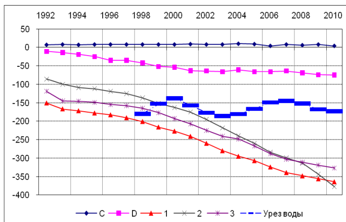
Рис.1. Динамика просадок поверхности на площадке 2 на участке Юкэчи
