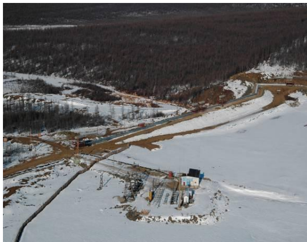
Рис. 9. Плотина на реке Лиендокит. Нюрбинский ГОК АК «Алроса»
