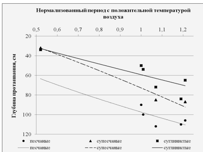
Рис. 2. Зависимость средней для участка глубины протаивания на песчаных, супесчаных и суглинистых породах от нормированной длительности теплого периода (точки измерения и степенная аппроксимация) за 2007 и 2010 годы
