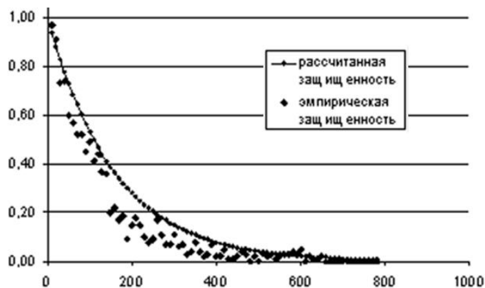
Рис. 4а. Сопоставление теоретических и эмпирических значений защищенности от термокарстовых процессов для линейного объекта разной протяженности (протяженность в пикселях - ось абсцисс, защищенность - ордината) до учета слияния озер.
