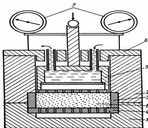
Рис. 4. Схема одометра
