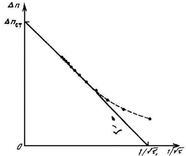
Рис. 2. График зависимости показаний гальванометра \Delta n (дел) от параметра 1/\sqrt{\tau} (c^{-1/2})
