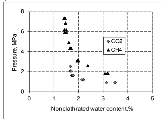
Рис. 3. Изменение содержания неклатратной воды в зависимости от газового давления CO_2 и CH_4 в каолиновой глине при -7,5^\circ C
