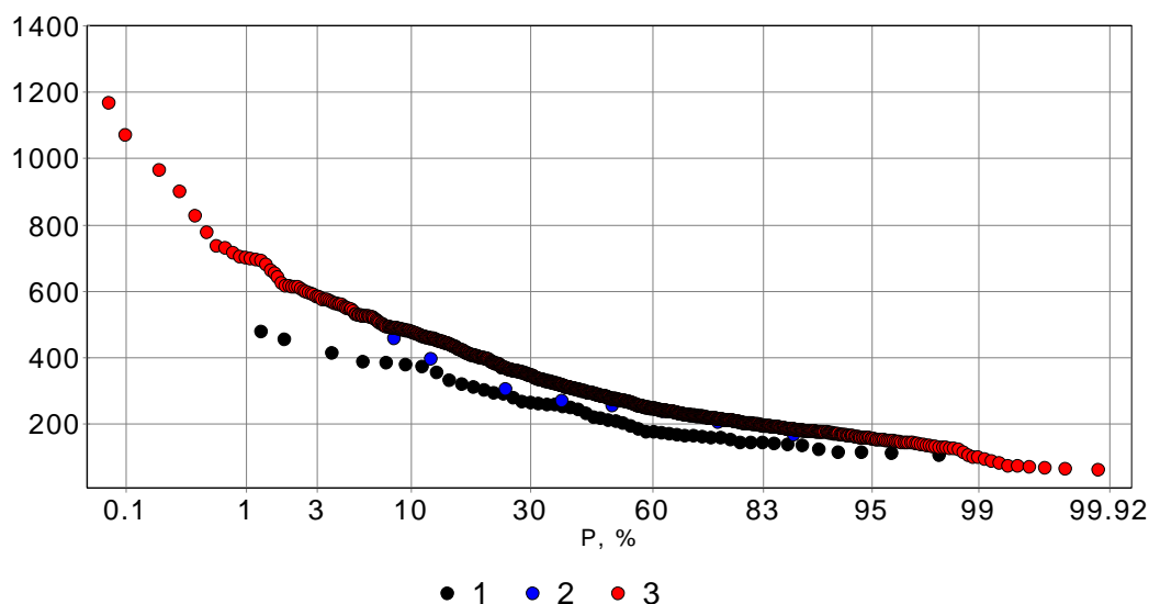
Рис. 4. Кривые распределения рассчитанных и наблюдаемых максимальных расходов воды ( \text{м}^3/\text{с} ) в бассейне р. Тенке, 2,2 км от устья р. Нилькоба (обозначения 1, 2, 3 – см. в тексте)
