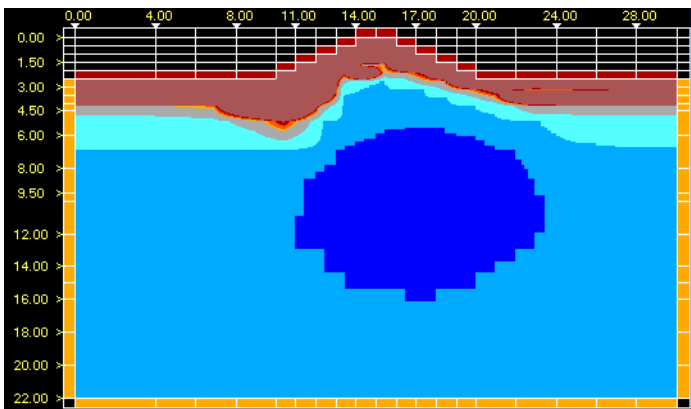
Рис. 5. Распределение температуры грунта через 30 лет после возведения насыпи (на 1 октября, когда оттаивание максимально).
