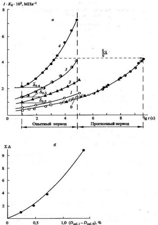
Рис. 4. Семейство кривых податливости мерзлого суглинка, засоленного NaCl при одноосном сжатии ( \sigma = 1,26 МПа), температуре -5^\circ\text{C} (а) и зависимость \Sigma \lg a_{D_{sal}} - (D_{sal,i} - D_{sal,0}) (б) при различной степени засоленности D_{sal} : 0-0%; 1-0,2; 2-0,4; 3-0,7; 4-1,5%
