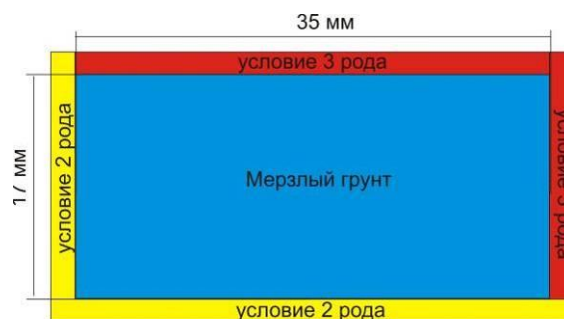
Рис 2. Пример разбивки расчетной области
