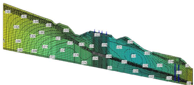
Рис. 6. Изолинии горизонтальных перемещений элементов в сооружении, м
