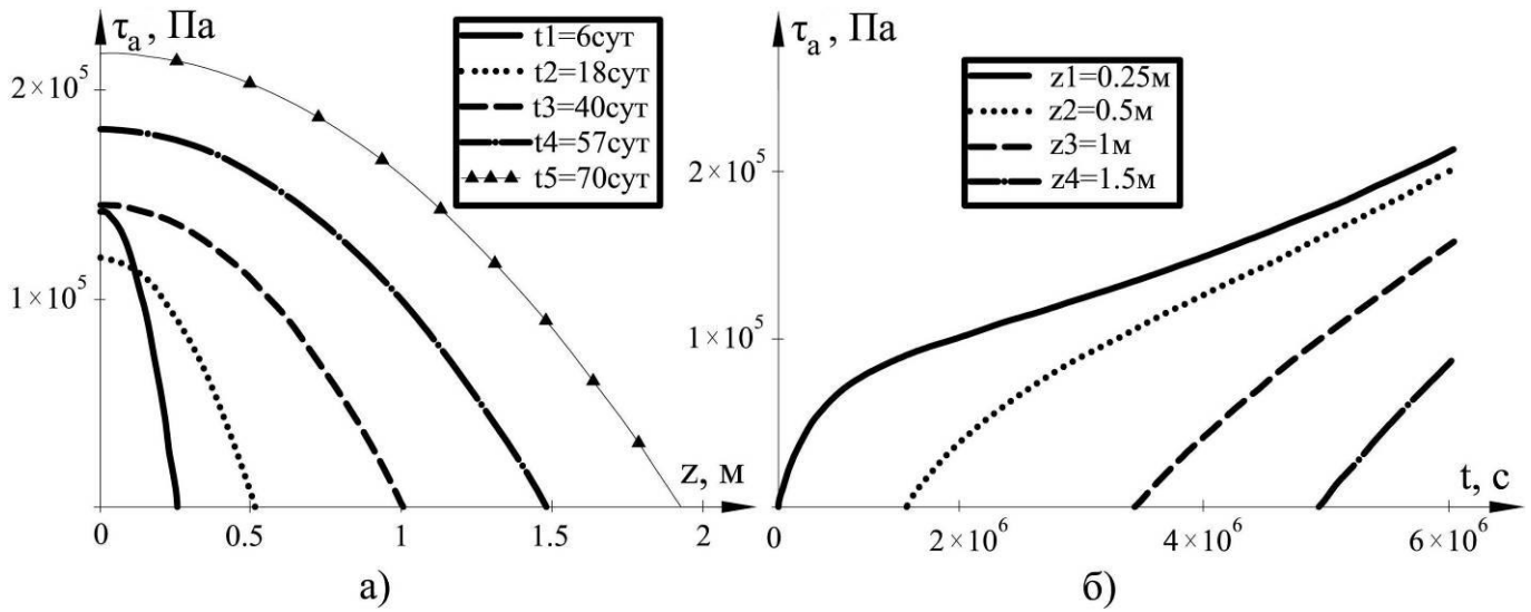
Рис.4. Графики зависимости касательного напряжения \tau_a при \eta(\theta)=const и \beta(t) : а) от координаты z для постоянных моментов времени t_1-t_5 ; б) от времени t для точек, расположенных на различных глубинах z_1-z_4
