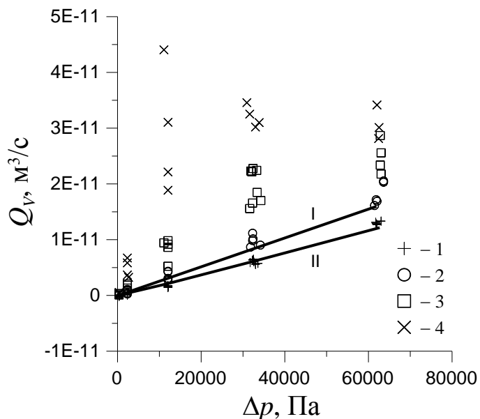
Рис. 2. Зависимость объемного потока жидкости Q_v через образец в зависимости от разности давлений \Delta p на границах образца при различных средних температурах t_0 . Символы – экспериментальные данные при различных средних температурах: -0,04 (1), -0,03 (2), -0,02 (3), -0,01 (4); линии – результат расчета при различных перепадах температуры на латунных пластинах: I - нулевом, II - максимальном из опытных данных (рис.3)
