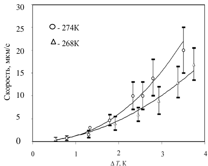
Рис. 5. Скорость роста корки метастабильных гидратов пропана на поверхности капель переохлажденной воды как функция переохлаждения и температуры
