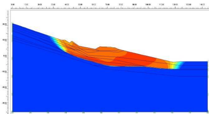
Рис. 3. Результат расчёта устойчивости сооружения на косогоре
