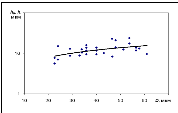
Рис.3. Величина зазора между каплями и поверхностью воды в зависимости от диаметра капли. Сплошная кривая ( h_0 ) – расчет из условия стоксо-гравитационного равновесия, маркеры ( h ) – результаты опытов
