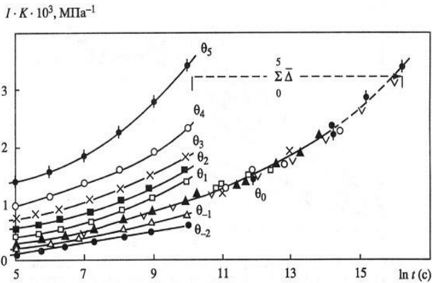
Рис. 2. Опытные кривые податливости и обобщенная прогнозная кривая для пушицево-сфагнового торфа (вдавливание шарикового штампа) при различной температуре: \theta_1 = -9,5^\circ\text{C} ; \theta_2 = -8,5 ; \theta_3 = -6 ; \theta_4 = -4 ; \theta_5 = -2,5 ; \theta_0 = -13 ; \theta_{-1} = -25,5 ; \theta_{-2} = -28^\circ\text{C}
