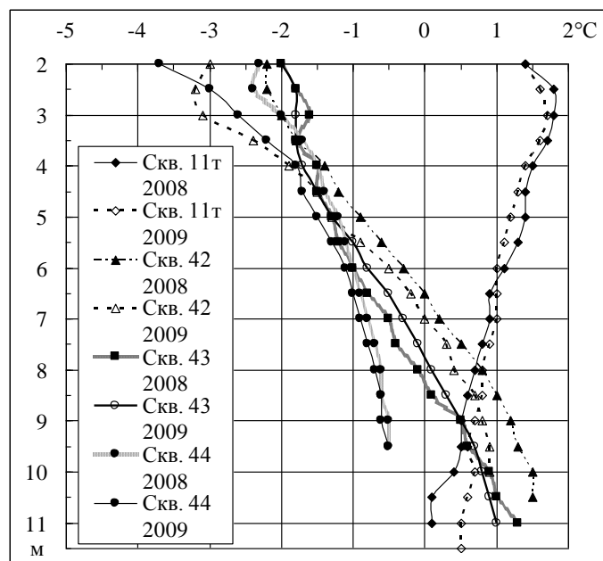
Рис. 11. Средние годовые температуры грунтов около УКЦ (скв. 11т) и вокруг здания химводоочистки.
