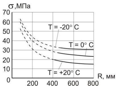
Рис.4. Изменение напряжений при изгибе трубы из полиэтилена ПЭ80 диаметром 63 мм (--- - недопустимые напряжения; — - допустимые напряжения)
