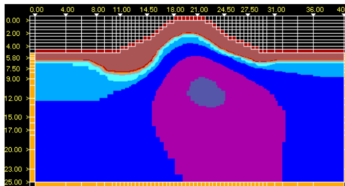
Рис. 7. Распределение температуры грунта через 10 лет после возведения насыпи (на 1 октября, когда оттаивание максимально).
