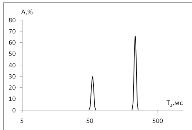
Рис.3. Распределение T_2 для оттаявшей дисперсии лед армированный ПВС/аэросил. Температура 30^\circ\text{C} .
