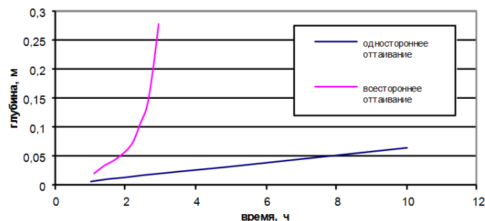
Рис 3. Зависимость глубина оттаивания от времени оттаивания
