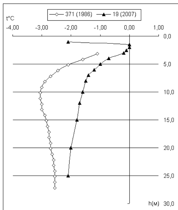
Рис. 3. Динамика температуры грунтов на левом берегу р. Щучьей в 1986-2007 г.г.
