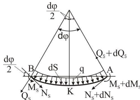
Рис.3. Элемент стержня
