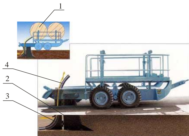
Рис.1. Общий вид трубоукладчика
