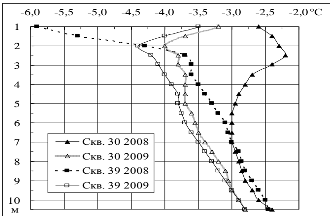
Рис. 5. Средние годовые температуры грунтов около западного угла главного корпуса.
