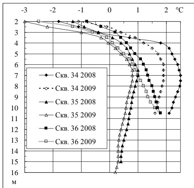
Рис. 10. Средние годовые температуры талых грунтов вокруг прибора к зданию водогрейных котлов.
