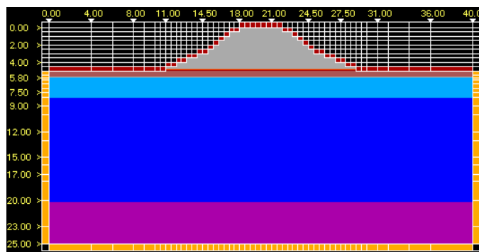
Рис. 6. Начальное распределение температурного поля (дата замера температуры – 18.09.08).
