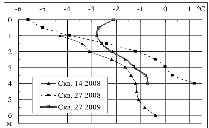
Рис. 7. Средние годовые температуры грунтов под главным корпусом вблизи таликовой зоны.
