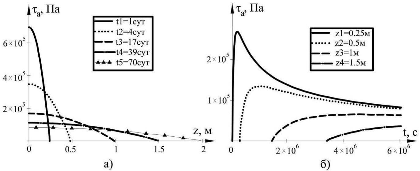
Рис.5. Графики зависимости касательного напряжения \tau_a при \eta(\theta)=const и \beta(t)=const : а) от координаты z для постоянных моментов времени t_1-t_5 ; б) от времени t для точек, расположенных на различных глубинах z_1-z_4
