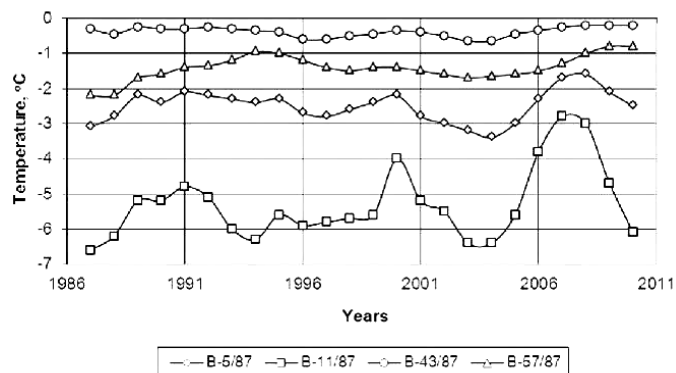
Рис. 2. Многолетняя изменчивость среднегодовой температуры грунтов на глубине 10 м, в различных типах местности: межгрядово-низинный (B-5/87), мелкодолинный (B-11/87), низкотеррасовый (B-43/87) и межгрядовый (B-57/87).
