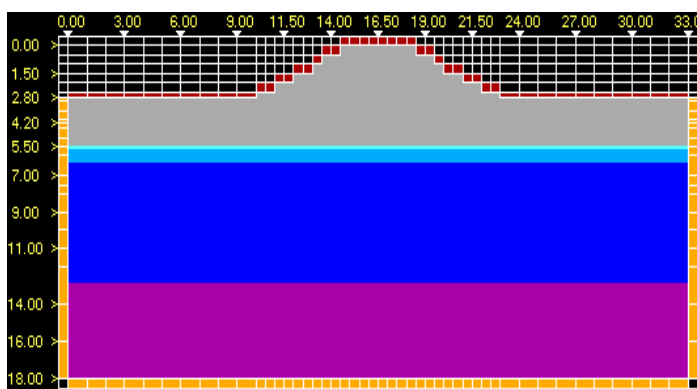
Рис. 9. Начальное распределение температурного поля (дата замера температуры – 18.09.08).
