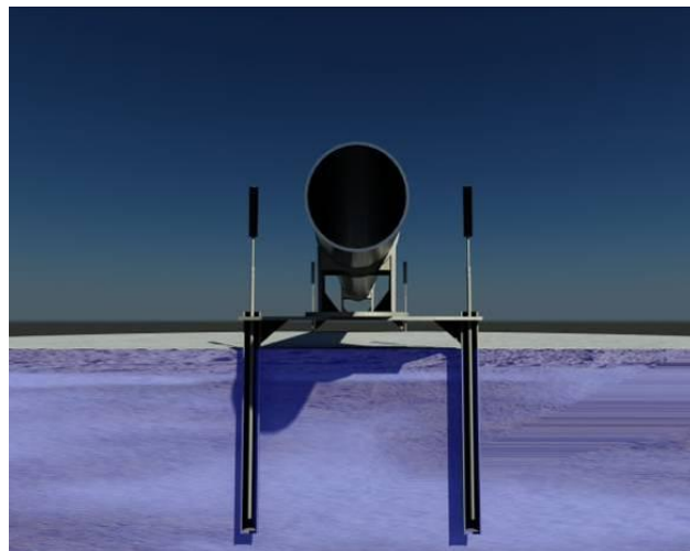
Рис. 7. Индивидуальные термостабилизаторы, установленные совместно со сваями
