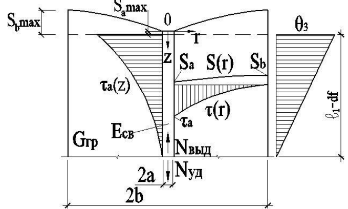
Рис. 2. Цилиндрическая геомеханическая модель взаимодействия сваи с промерзающим пучинистым грунтом
