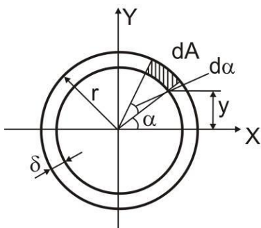
Рис.2. Схема поперечного сечения трубы (dA – элементарный участок сечения, r – радиус трубы, delta – толщина стенки трубы)
