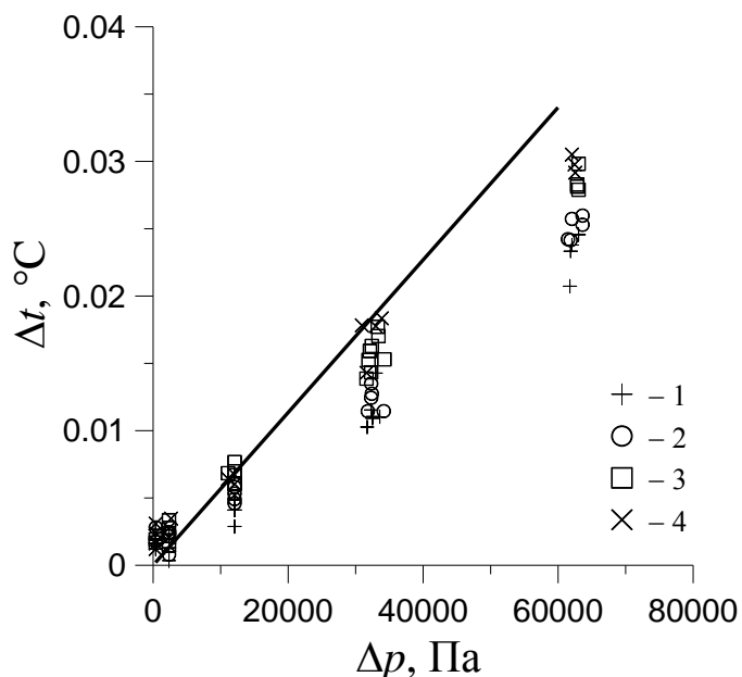
Рис. 3. Разность температур \Delta t между основаниями образца (латунные пластины 2, рис.1) в зависимости от перепада давления жидкости \Delta p . Символы – экспериментальные данные при различных средних температурах: -0,04 (1), -0,03 (2), -0,02 (3), -0,01 (4); линия – результат расчета.
