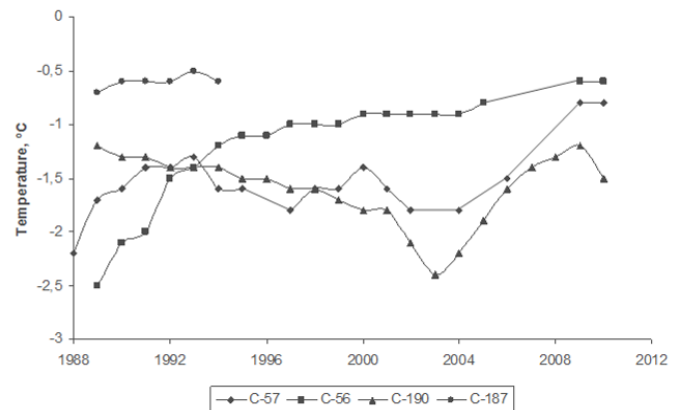
Рис. 3. Динамика среднегодовой температуры грунтов в лиственничнике (С-57), при выборочной (С-187), постепенной (С-56) и сплошной (С-190) рубках леса в межгалазье.
