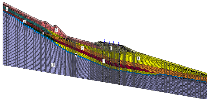
Рис. 1. Расчетная схема конструкции 1 – насыпной грунт; 2 – песок гравелистый талый маловлажный; 3 – суглинок легкий с дресвой до 20%, маловлажный; 4 – суглинок тяжелый пылеватый с дресвой до 20%, мягкопластичный; 5 – суглинок легкий с дресвой до 10%, тугопластичный, с прослойками песка влажного; 6 – супесь легкая с дресвой до 20%, твердая; 7 – суглинок дресвяный твердый; 8 – суглинок тяжелый с дресвой до 10%, мерзлый, слабольдистый, массивной криотекстуры; 9 – прослойка оттаявшего мерзлого грунта; 10 – вечномерзлый грунт
