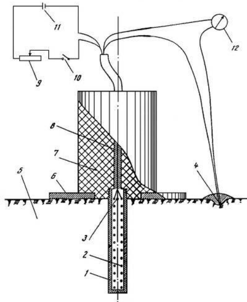
Рис. 3. Схема конструкции короткого цилиндрического зонда
