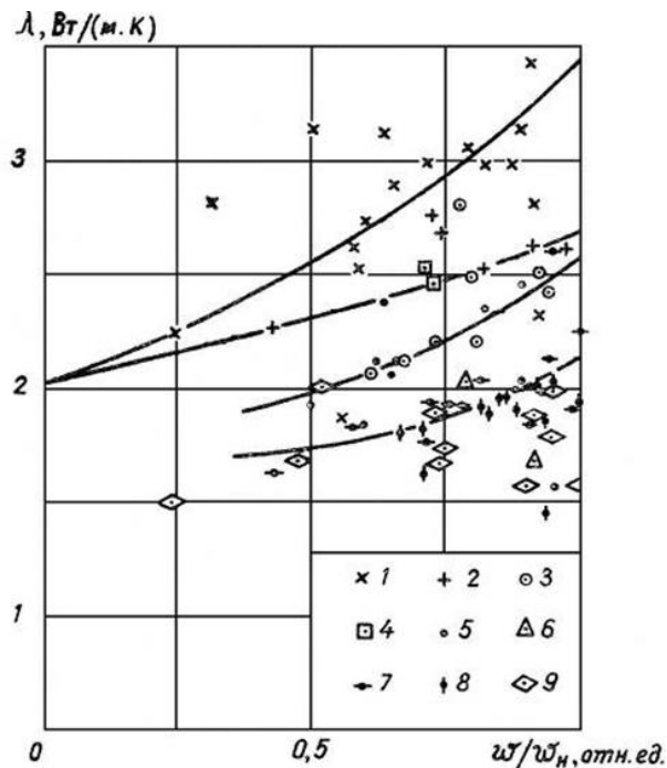
Рис. 4. Коэффициент теплопроводности массива горных в штольне №1000 в зависимости от степени влагонасыщения для различных типов пород:
