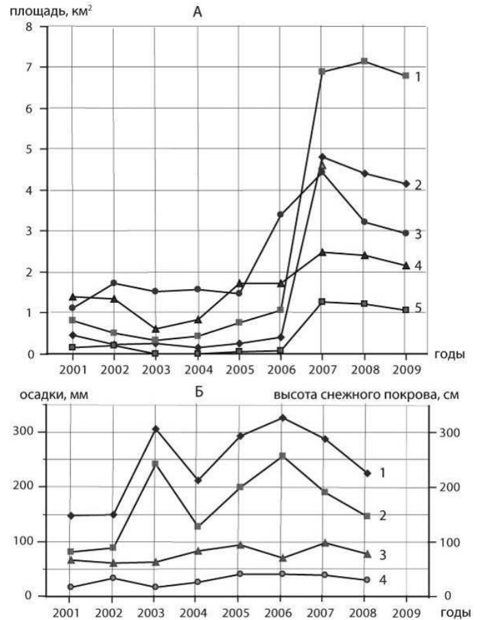
Рис. 9. Графики годовых изменений площади отдельных крупных озер (А): 1 – Тюнъюлю, 2 – Сегелей, 3 – Нал-Тюнъюлю, 4 – Абалах, 5 – Майя. Ход метеорологических характеристик (Б): 1 – среднегодовые осадки, 2 – летние осадки, 3 – зимние осадки, 4 – высота снежного покрова
