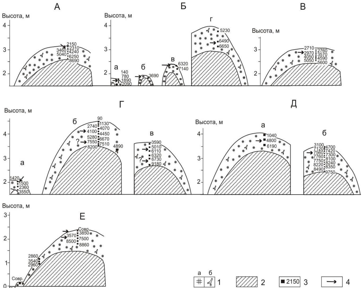
Рис. 2. Радиоуглеродное датирование бугров пучения в Большеземельской тундре [uz Vasil'chuk et al. 2003, 2008]: А - пос. Бугры, Б - пос. Уса, В - пос. Абезь, Г - пос. Никита, Д - пос. Елецкий, Е - пос. Хановей. 1 – материал датирования торф (а) и ветки деревьев (б), 2 – суглинок, 3 – радиоуглеродные датировки, 4 – момент пучения
