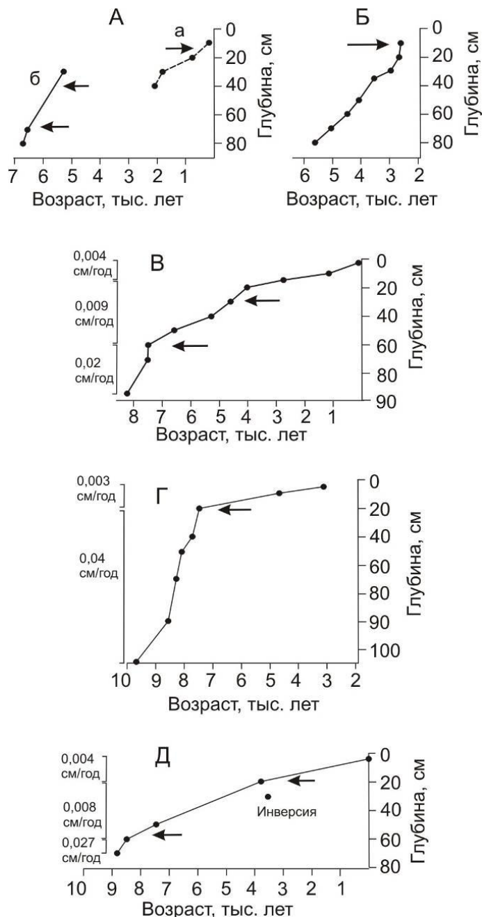
Рис. 3. Предполагаемые моменты пучения (показаны стрелками) и скорость торфонакопления в буграх пучения в Большеземельской тундре: А - пос. Уса, Б - пос. Абезь, В - пос. Никита, Г - пос. Елецкий, Д - пос. Хановей
