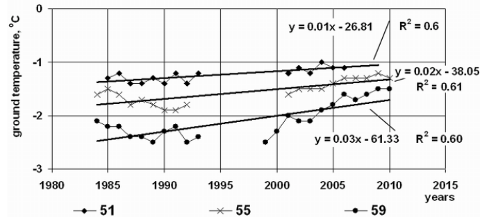
Рис.12. Временная изменчивость среднегодовой температуры пород в различных ландшафтных условиях на стационаре Болванский: скв. 59 – типичная тундра; скв. 55 – деградирующий полигональный торфяник; скв. 51 – дренированная тундра на бровке озера
