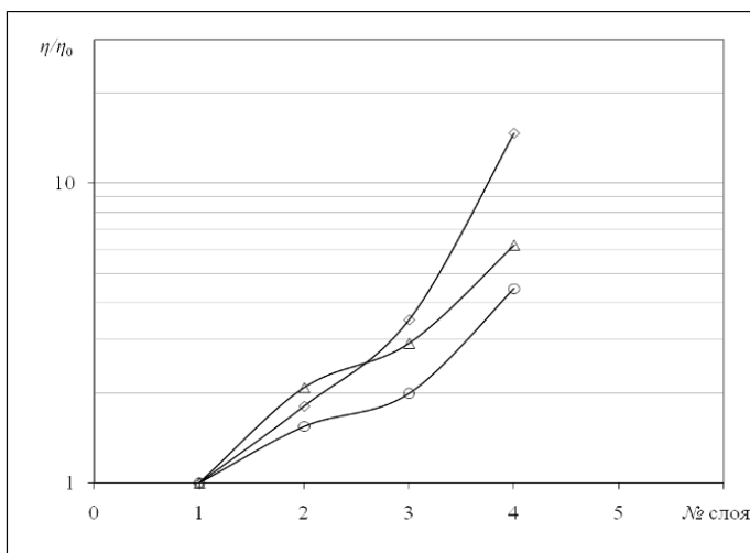
Рис.5. Коэффициент двиговой вязкости \eta в различных слоях кластера при температуре 90°C. \eta_0 –вязкость воздуха
