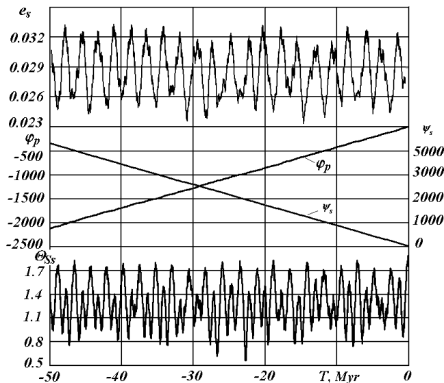
Рис. 3. Эволюция параметров орбиты Земли за -50 млн. лет в прошлое: e_s - скользящие средние эксцентриситета; \varphi_p - угол перигелия; \psi_s - угол прецессии; \theta_{ss} - скользящие средние угла нутации оси орбиты. Углы \varphi_p и \psi_s даны в радианах, \theta_{ss} - в градусах. Myr - млн. лет.
