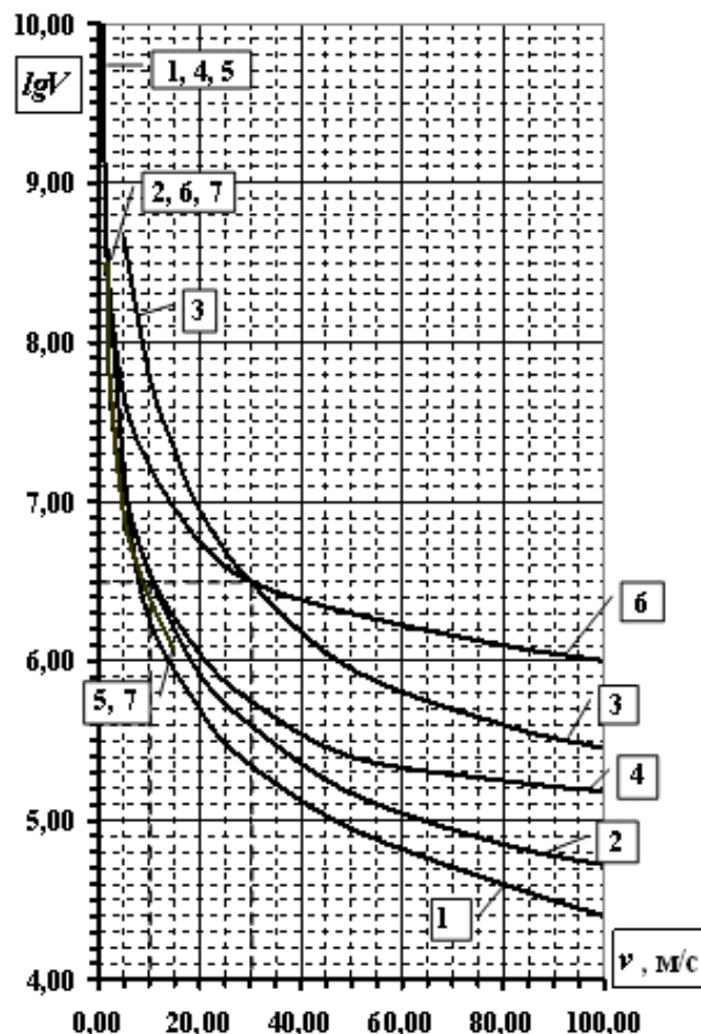
Рис.1. Расчётные критерии катастрофического протекания экзогенных геологических процессов. Вертикальная ось – логарифм объёма перемещаемого материала, \text{м}^3 ; средняя скорость перемещения материала, м/с: 1 – обвалы; 2 – трещинообразование; 3 – дефляция – перевывание; 4 – сели; 5 – оползни; 6 – снежные лавины; 7 – криогенные сплывы
