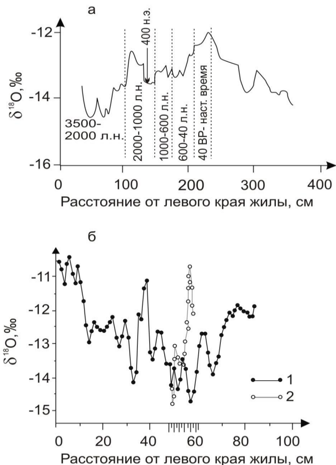
Рис.4. Вариации \delta^{18}O в голоценовых жилах в долине Адвентдален: а) по J.W.Jeppesen [2001], б) по H.Vittinghus et al. [2008]. 1 – жила нижнего яруса, 2 – жила верхнего яруса, внедряющаяся в нижнюю жилу.
