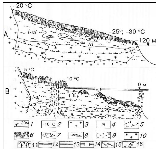
Рис. 5. Строение шельфа моря Лаптевых [Романовский и др. 1997].
