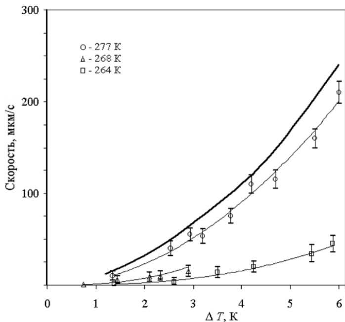
Рис.4. Скорость роста гидратов метана на поверхности капель воды как функция переохлаждения и температуры. Жирная линия представляет степенной тренд по литературным данным для скорости роста стабильных гидратов на поверхности объемной воды
