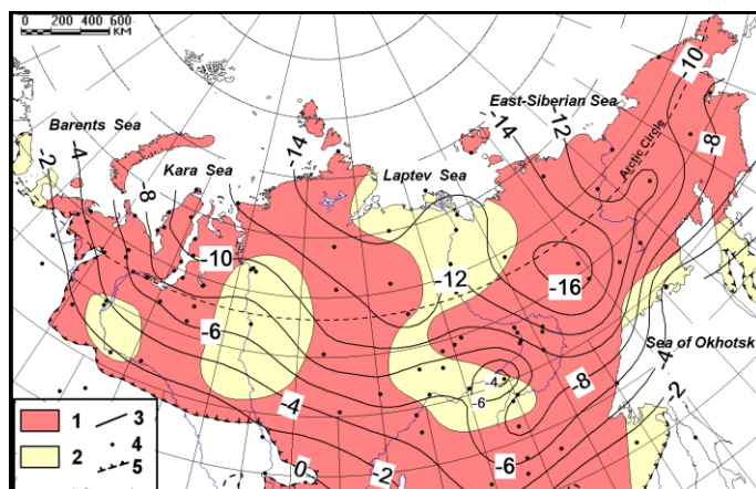
Рис. 1. Изменчивость среднегодовой температуры воздуха Условные обозначения: повышение температуры в последнее десятилетие относительно нормы: 1 - сильное, \Delta t > 1,0^{\circ}\text{C} ; 2 - умеренное, 0,7 \leq \Delta t \leq 1^{\circ}\text{C} ; 3 - изолинии среднегодовой температуры воздуха (норма); 4 - метеостанции; 5 - южная граница криолитозоны
