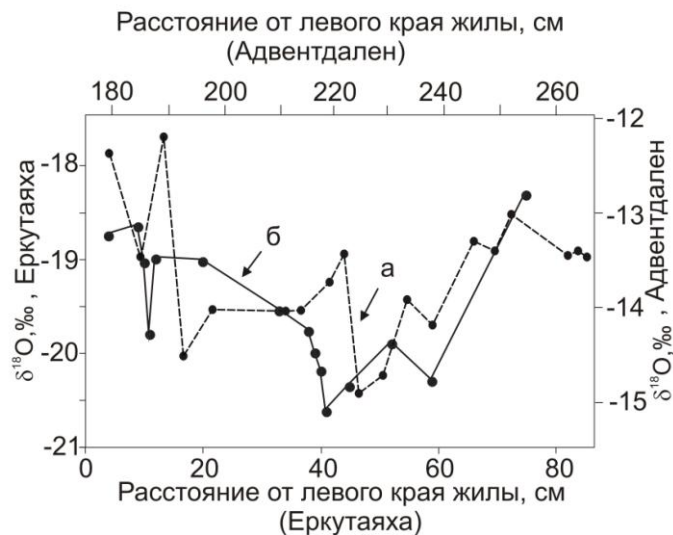
Рис. 5. Сопоставление фрагментов изотопной записи по жильному льду в долине Адвентдален (а) и на пойме р.Еркутаяха (б)
