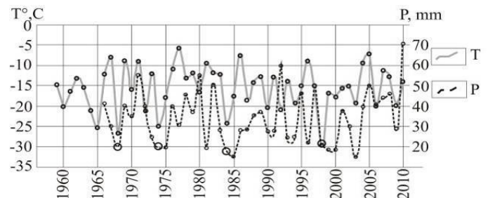
Рис.7. Изменение количества атмосферных осадков в ноябре (P, mm) и температуры воздуха (T, °C)
