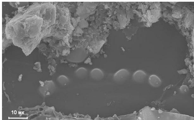
Рис.1. Расположение клеток микроорганизмов в штире сегрегационного льда суглинков Мамонтовой горы.
