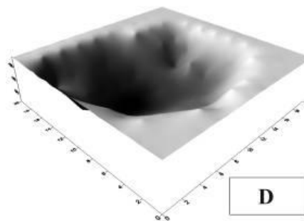
Рис. 10. Старая термокарстовая западина в 2005 (А), 2010 (В) и 2011 (С) г., объемное изображение понижения в 2009 г, полученное в программе «Surfer» (D)
