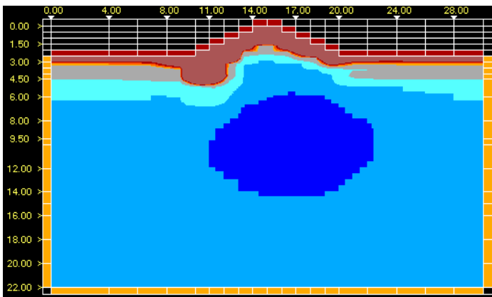
Рис. 4. Распределение температуры грунта через 10 лет после возведения насыпи (на 1 октября, когда оттаивание максимально).
