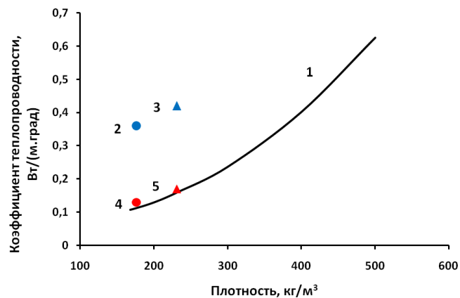
Рис. 4. Коэффициенты теплопроводности: 1 - снега; 2 и 4 - мох H. splendens var alascanum ; 3 и 5 - мох S. uncinata ; 2 и 3 - зимой; 4 и 5 - летом
