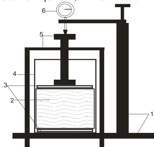
Рис 5. Схема компрессионного прибора 1 – станина; 2 – металлическое кольцо с грунтом; 3 – перфорированные штампы; 4 – внешний цилиндр; 5 – система рычагов для подачи нагрузки; 6 – индикатор.
