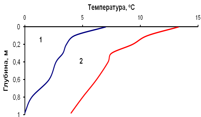
Рис. 1. Температура грунта: 1 - под моховым покровом толщиной 8 см; 2 - без мохового покрова
