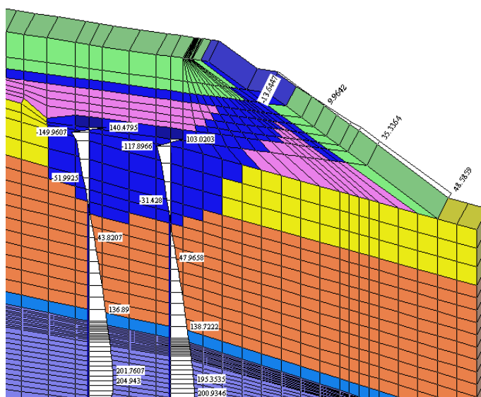
Рис. 5. Эпюры горизонтальных напряжений свайной конструкции, кПа
