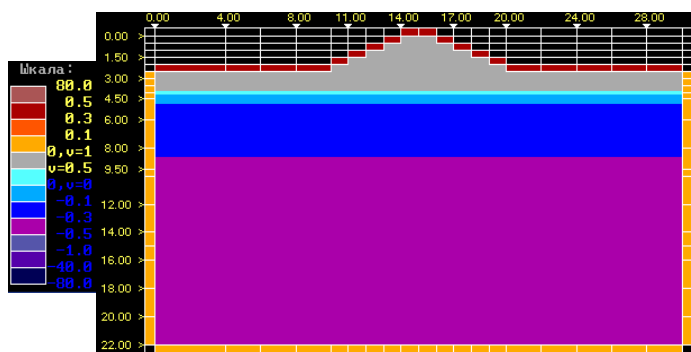
Рис. 3. Начальное распределение температурного поля (дата замера температуры – 30.04.08)
