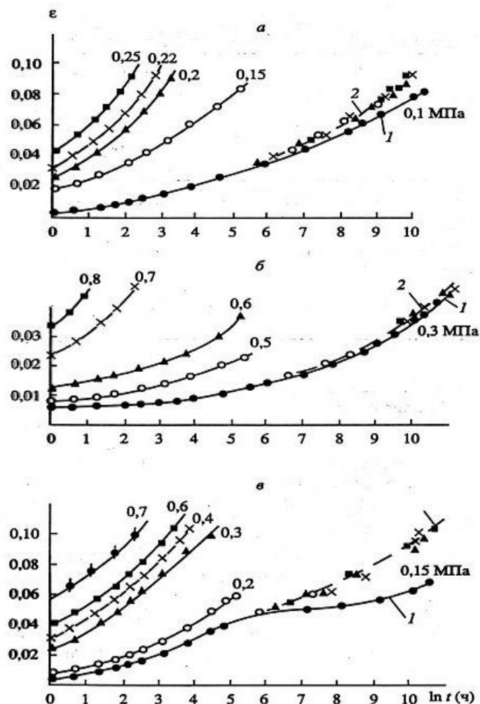
Рис. 5. Кривые ползучести мерзлых грунтов (одноосное сжатие) 1 – опытные данные А.В.Брушкова, 2 – прогнозные данные по методу напряженно-временной аналогии; а – суглинок; б – супесь, в – песок.
