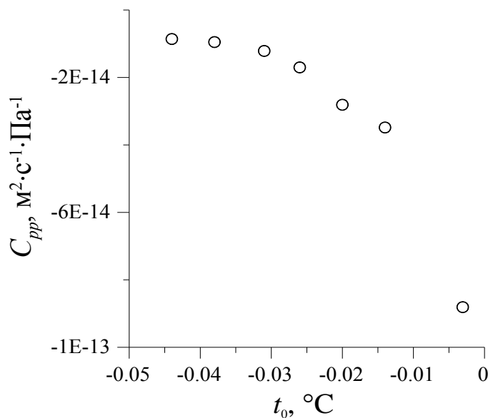
Рис. 5. Зависимость коэффициент C_{pp} от средней температуры образца
