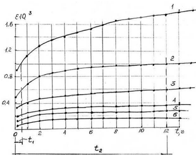
Рис.1. Кривые ползучести \epsilon мерзлого суглинка (одноосное сжатие, температура \theta = -40^{\circ}\text{C} ) при различном напряжении \sigma , МПа: 1-1.2; 2-1.0; 3-0.8; 4-0.5; 5-0.36; 6-0.2.
