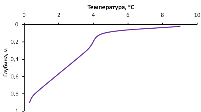
Рис. 2. Распределение температуры во мху толщиной 8 см и в грунте
