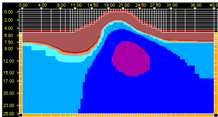
Рис. 8. Распределение температуры грунта через 30 лет после возведения насыпи (на 1 октября, когда оттаивание максимально)
