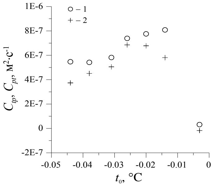
Рис. 7. Зависимость недиагональных коэффициентов переноса C_{IP} (1) и C_{PI} (2) от средней температуры образца
