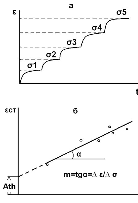
Рис.6. Зависимости развития относительной осадки от времени при каждой ступени нагружения (а), условно- стабилизированной осадки - от напряжения (б)
