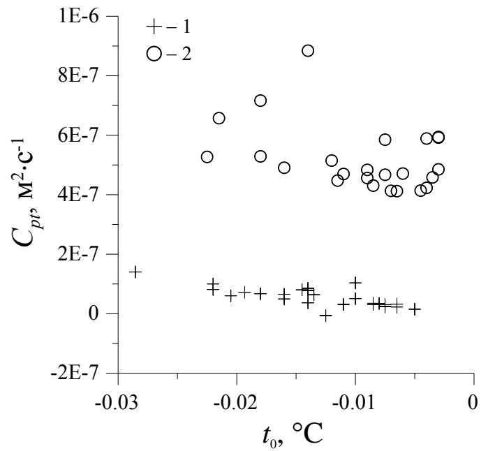
Рис. 8. Зависимость коэффициента переноса C_{PI} от средней температуры образца для 1 и 2 серий измерений
