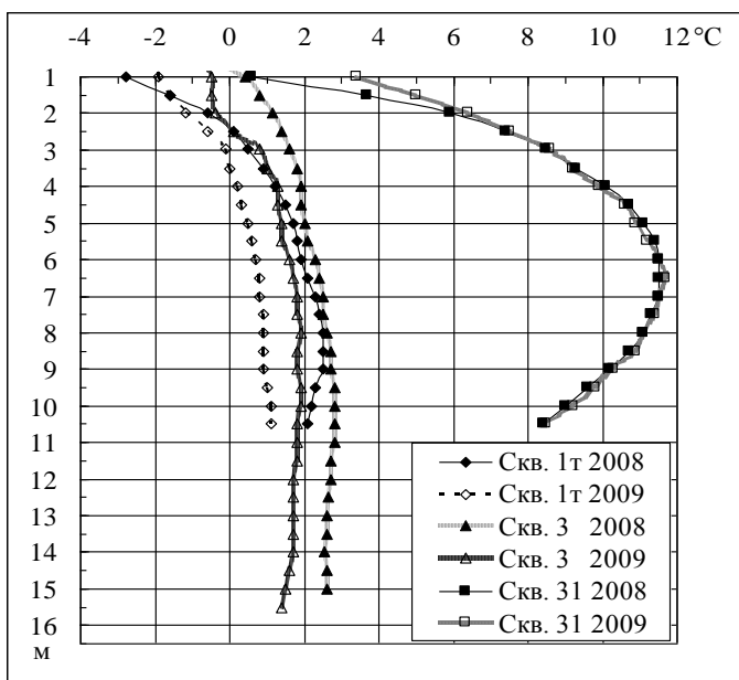
Рис. 8. Средние годовые температуры грунтов в таликовой зоне вокруг циркуляционной насосной станции.
