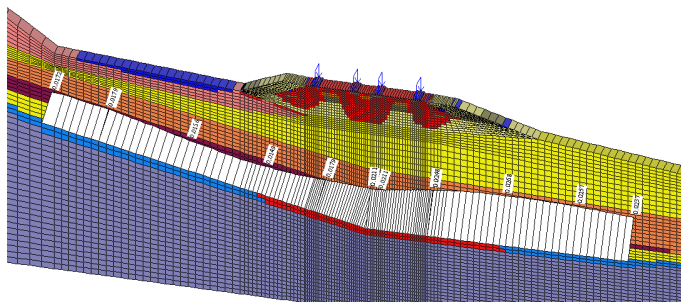
Рис. 2. Зоны упругих (синий цвет) и пластических (красный цвет) деформаций и эпора горизонтальных перемещений грунтового массива в зоне прослойки оттаявшего мерзлого грунта, м
