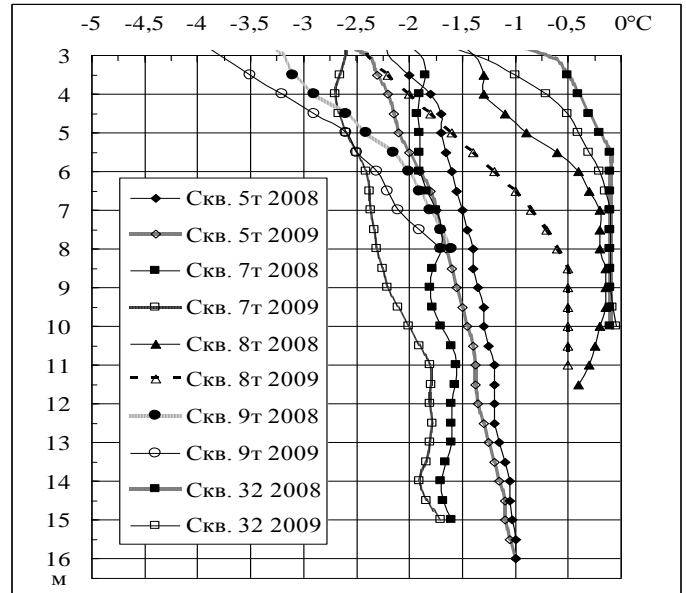
Рис. 6. Средние годовые температуры грунтов вокруг основной части главного корпуса.
