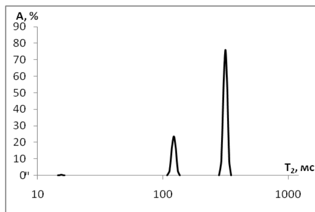
Рис.2. Распределение T_2 для оттаявшей дисперсии “чистый” лед/аэросил. Температура 30^\circ\text{C} .
