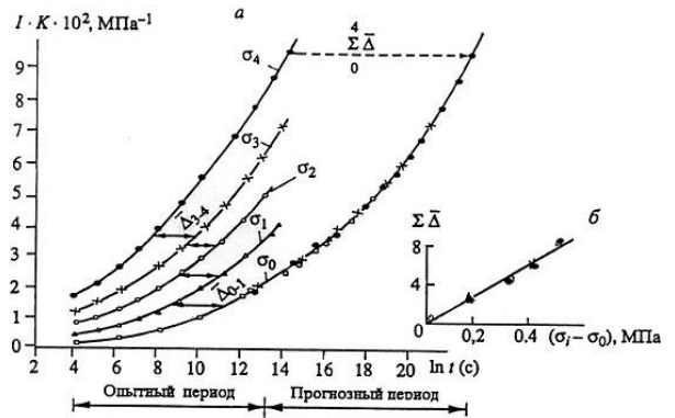
Рис. 3. Семейство кривых податливости для мерзлого верхового пушицево-сфагнового торфа при одноосном сжатии, температуре -4,5^\circ\text{C} и различном напряжении (а) \sigma_0 = 0,2 МПа; \sigma_1 = 0,36 ; \sigma_2 = 0,5 ; \sigma_3 = 0,6 ; \sigma_4 = 0,7 и зависимость \Sigma \Delta \ln a_{\sigma} - (\sigma_i - \sigma_0) (б)
