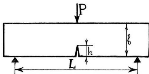
Рис.1. Схема нагружения образца.
