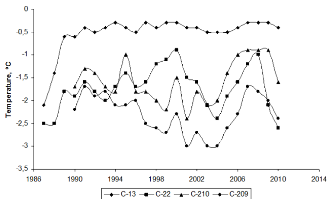
Рис. 4. Динамика среднегодовой температуры грунтов в сосняке (С-22), на гари с вырубкой (С-13), в песчано-грядовом и в лиственничнике (С-210), на гари с вырубкой (С-209) в межлассном типе местности
