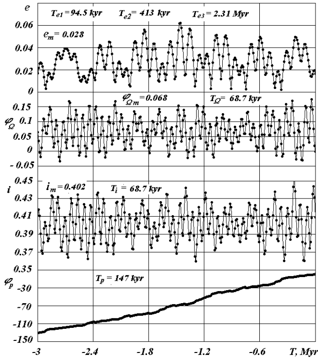
Рис. 2. Эволюция орбиты Земли за 3 млн. лет в прошлое: e - эксцентриситет; \varphi_Q - угловое положение восходящего узла плоскости орбиты; i - угол ее наклона к неподвижной плоскости экватора; \varphi_p - угловое положение перигелия; T - время в миллионах лет от 1950 г. Углы даны в радианах.
