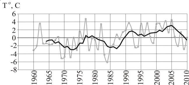
Рис.4. Изменения среднемесячной температуры воздуха в мае (T, °C) и линия тренда (пятилетняя скользящая)
