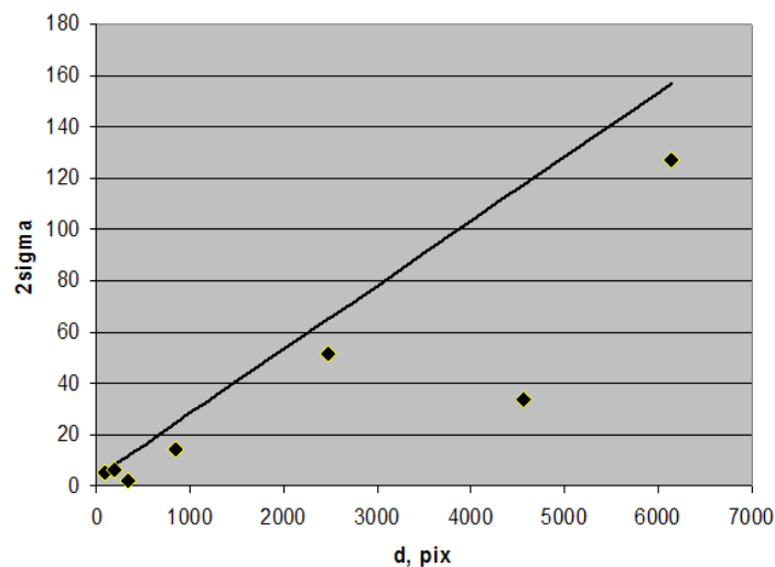
Рис. 3. График оценки ошибки дешифрирования для снимка 1987 г.
