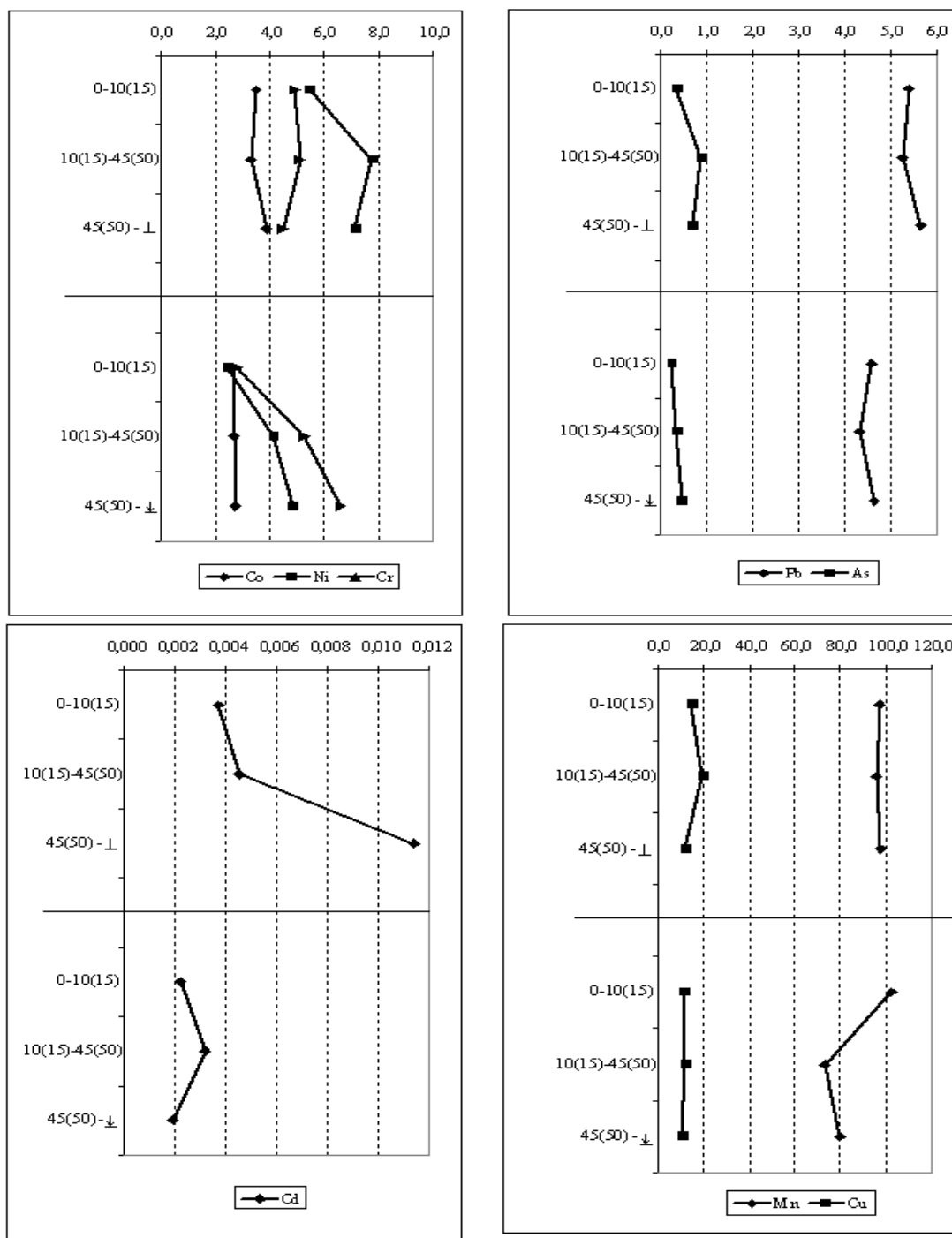
Рис. 2. Содержание подвижных форм микроэлементов в криоземах с присутствием «сухой» и «льдистой» мерзлоты ↑ - «льдистая» мерзлота; ↓ - «сухая» мерзлота
