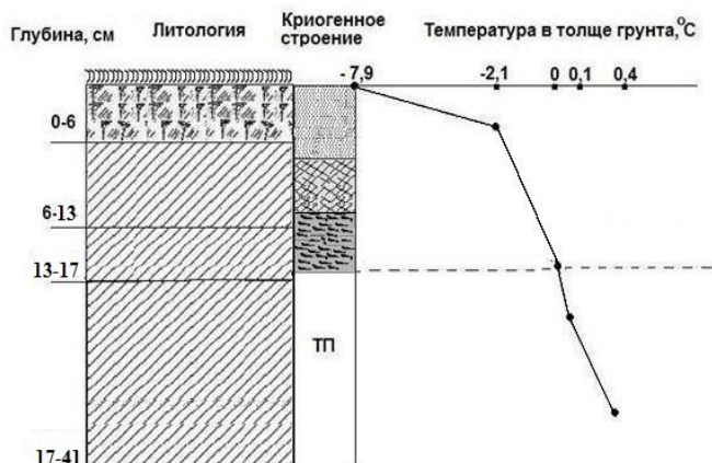
Рис.2. Литология, криогенное строение и температура грунта по профилю шурфа №4
