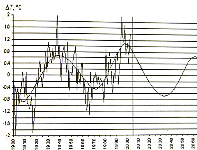
Рис. 3. Изменения аномалии среднегодовой температуры воздуха в широтной зоне 70-85° с.ш. в XX – начале XXI века и её фоновый прогноз [Фролов и др. 2007]
