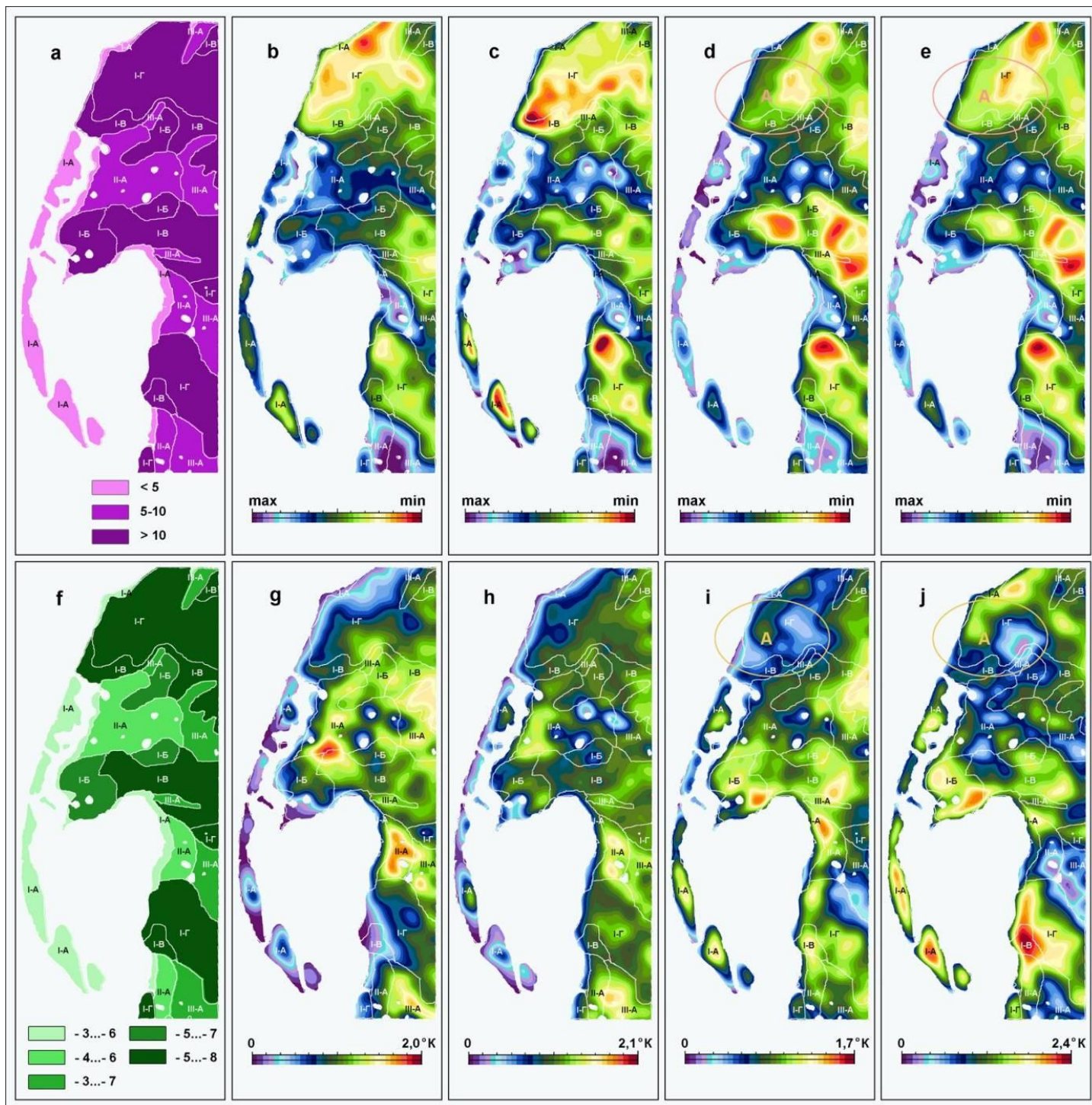
Рис. 2 Фрагменты карт макрольдистости грунтов в % (а), температуры ММП в °С (f) (Баулин et al. 2003), распределения параметров Е (b,c,d,e), СРТП (g,h,i) и разности СРТП (j) в районе Харасавэйского и Крузенштерновского ГКМ, полученных по данным съемки со спутника NOAA: 28 и 29 июня 2000 г. (b,g); 08 и 09 июля 2000 г. (c,h); 22 и 24 августа 1998 г. (d,i). Природные комплексы (Баулин et al. 2003): (I-A) – лайда; (I-B) – I морская терраса; (I-B) – II морская терраса; (I-Г) – III морская терраса; (II-A) – низовья крупных рек; (III-A) – пойма.
