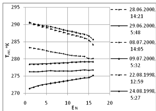
Рис. 1 Зависимость медианных значений радиационной ТП ( T_{rM} ) от «кажущейся тепловой инерции» ( E_N )
