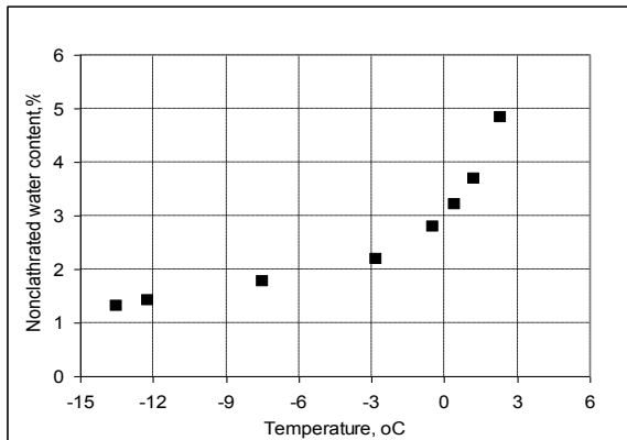
Рис. 2. Влияние температуры на содержание неклатратной воды в каолиновой глине под давлением CO_2 ( P = 1.6 МПа)
