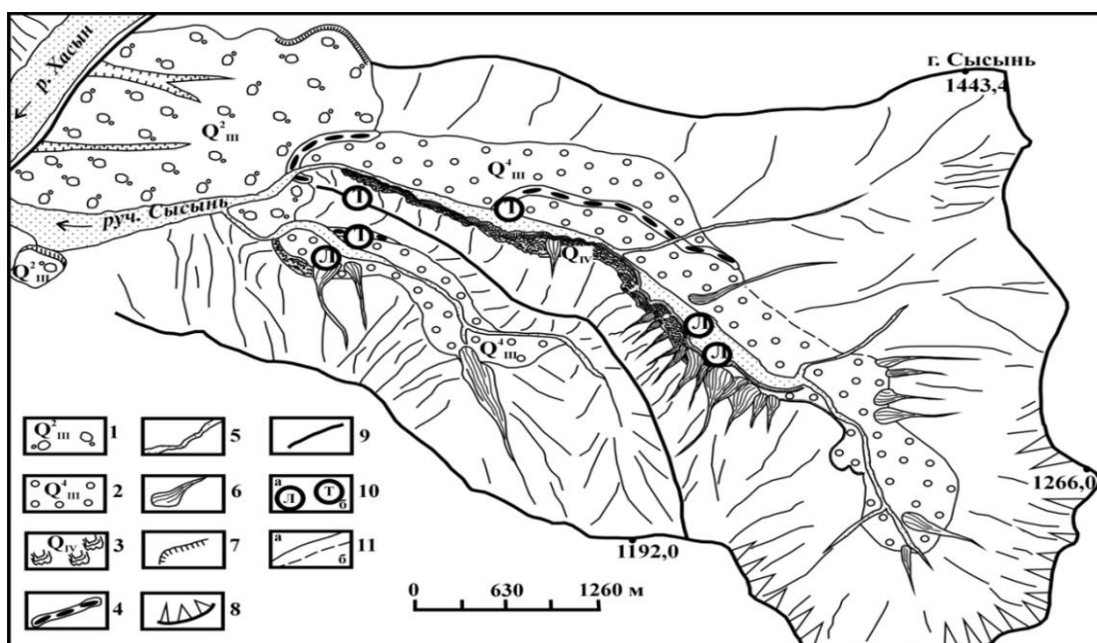
Рис. 4. Геоморфологическая схема каменного глетчера Карамкенский в верховьях ручья Сысынь (Хребет Дел-Урэчен):
