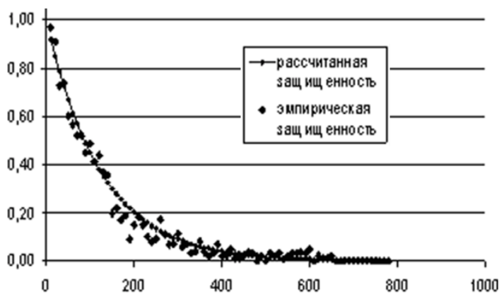
Рис. 46. Сопоставление теоретических и эмпирических значений защищенности от термокарстовых процессов для линейного объекта разной протяженности (протяженность в пикселях – ось абсцисс, защищенность – ордината) после учета слияния озер.
