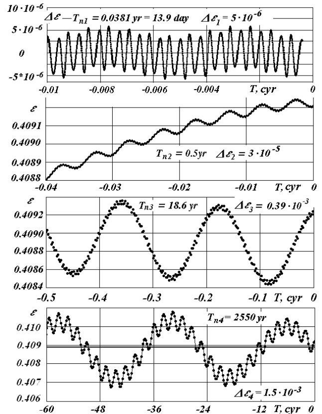
Рис. 5. Нутационные колебания оси вращения составной модели Земли No. 3 на разных интервалах времени: \Delta\varepsilon – отклонение угла нутации от скользящего среднего; \Delta\varepsilon_1, \Delta\varepsilon_2, \Delta\varepsilon_3, и \Delta\varepsilon_4 – амплитуды колебаний, 1 \text{cyr} = 100 лет. Углы даны в радианах.
