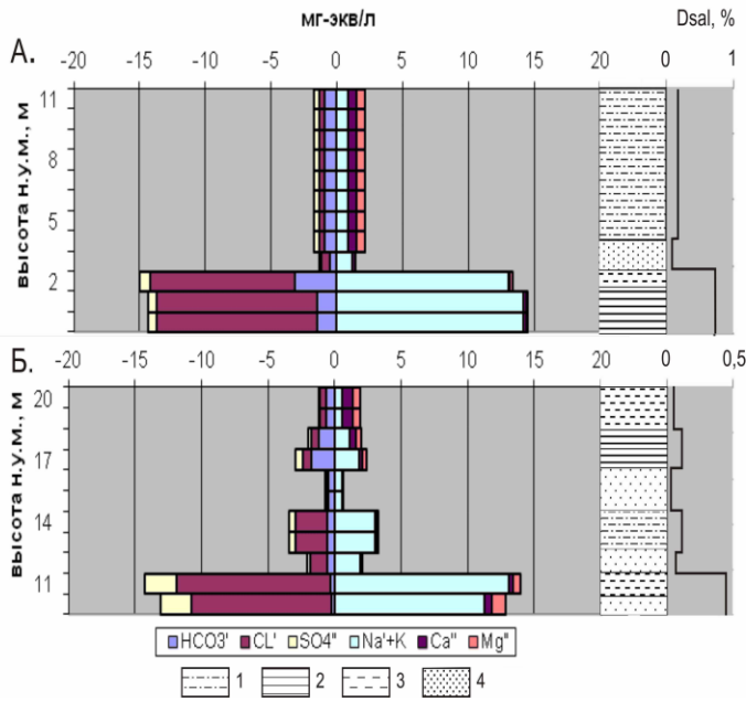
Рис. 3. Распределение ионов воднорастворимых солей в верхнеплейстоценовых песчано-глинистых отложениях Западного Таймыра: А. мыс Сопочная Карга; Б. устье р. Крестьянка. Со знаком минус на графике дано содержание анионов
