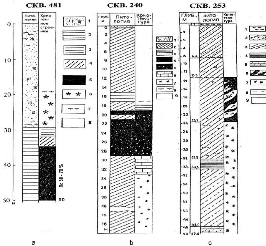
Рис.2. Разрез донных отложений на Баренцево-Карском шельфе [Мельников и Спесивцев 1995].
