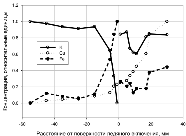
Рис. 2. Калий, медь и железо в тыльной и передовой зонах влияния включения сегрегационного льда
