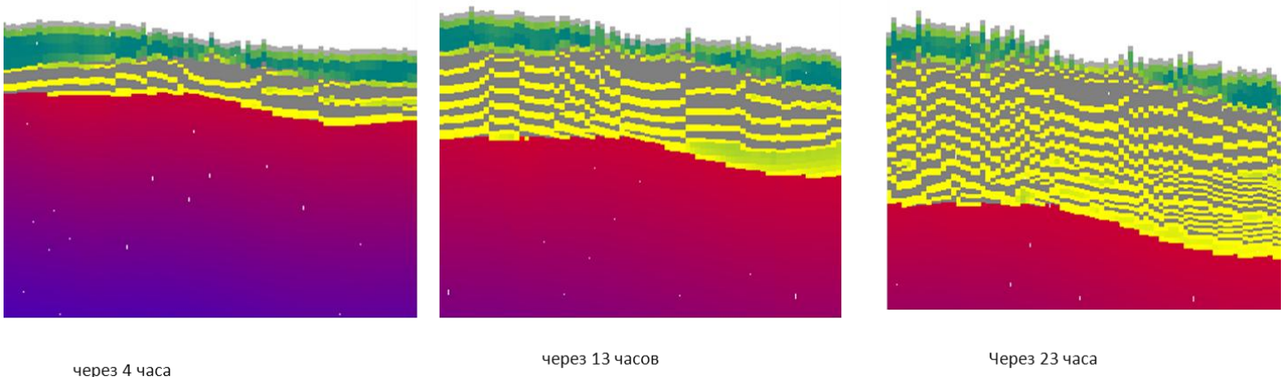
Рис. 3. Формирование криогенной текстуры промерзающей каолинитовой глины во времени. Талая зона отмечена красно-синим цветом, при этом реализована градация по влажности при переходе от красного цвета к синему в сторону увеличения влажности грунта. В качестве красного цвета изображен грунт с содержанием влажности предела усадки, а синим - предела текучести. Серым цветом обозначены прослои льда, а желто-зеленым мерзлые слои, льдистость которых возрастает от желтого к зеленому цвету.
