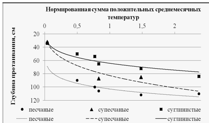
Рис. 3. Зависимость средней для участка глубины протаивания на песчаных, супесчаных и суглинистых породах от нормированной суммы температур теплого периода (точки измерения и степенная аппроксимация) за 2007 и 2010 годы
