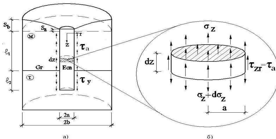
Рис. 1. Расчетная схема взаимодействия сваи с промерзающим пучинистым грунтом
